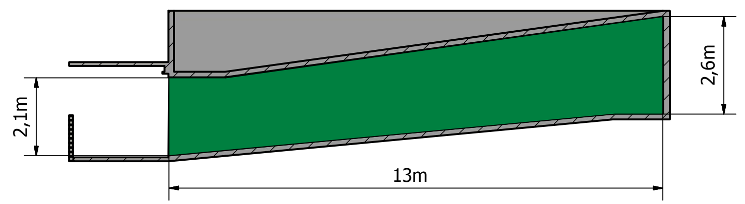
H-H ( 1 : 100 )
