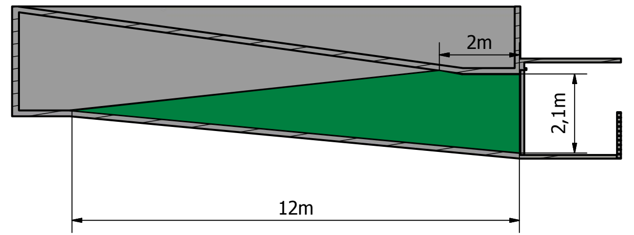
G-G ( 1 : 100 )
